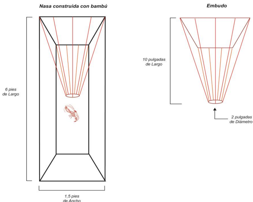
Fig. 3. Esquema ilustrativo de las artes de pesca utilizados para la captura de ejemplares del Genero Macrobrachium durante los muestreos.
