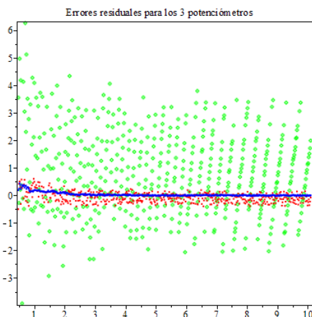
Figura 3. Errores residuales para las mediciones realizadas con los voltímetros digitales. Puntos verdes resolución de 1 mV, puntos rojos 0.1 mV y puntos azules 0.01 mV.
