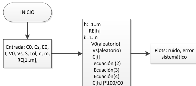
Figura 1. Esquema del programa de simulación del ruido aleatorio y el error sistemático de volúmenes de estándares adicionados a solución muestra de prueba.
