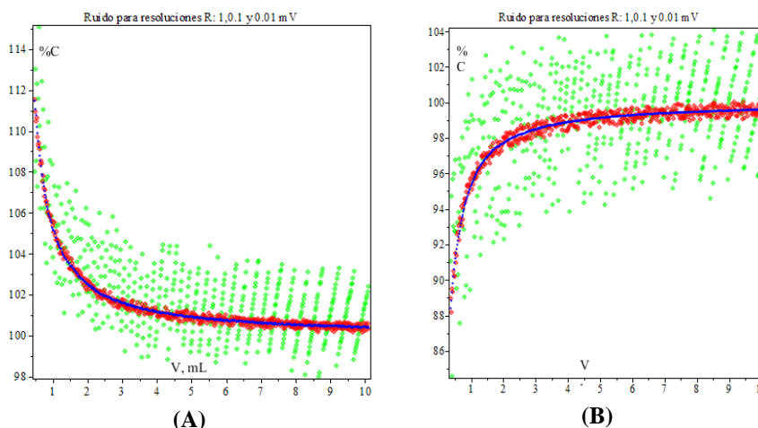
Figura 2. Ruido aleatorio y error sistemático expresado como porcentaje de concentración en función de volúmenes de estándar de cloruros adicionados. Los valores aleatorios de los potenciales son generados para 3 voltímetros digitales con resoluciones: a) 1 mV para los puntos verdes; b) 0.1 mV para los rojos; c) 0.01 mV para los azules. Gráficas: (A) desviación de 0.05 del valor nominal del volumétrico; (B) desviación negativa -0.05 del valor nominal.
