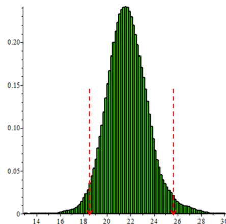
Figura 5. Histograma y límites de cobertura en la determinación de cloruros en agua de consumo humano.
